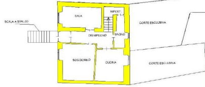
PIANTA PIANO TERRA
