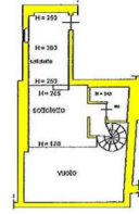
Piano secondo
