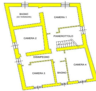
PIANO PRIMO h=2.60
