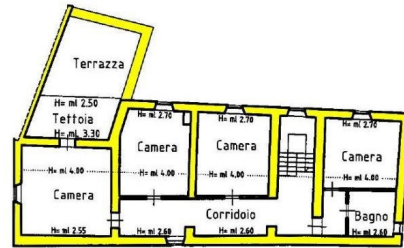
PIANO PRIMO
