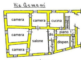
Piazza del Duomo -PIANTA PIANO PRIMO- h. s. 60
