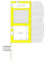
PIANTA SEMINTERRATO - scala 1:100
