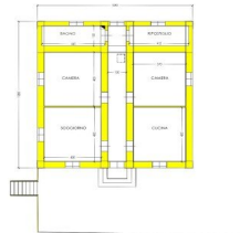
PIANTA PIANO TERRA
