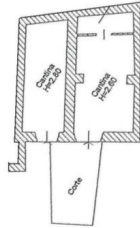
PIANO 1° SOTTOSTRADA
